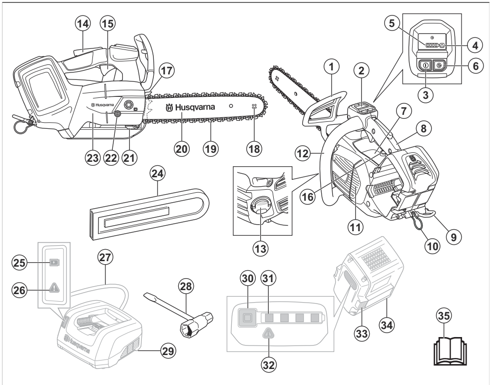
1. フロントハンドガードおよびチェンブレイキ
